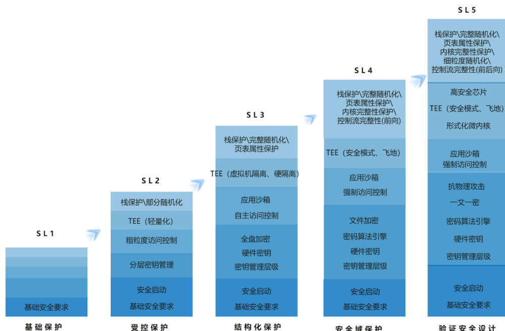
图5-2 HarmonyOS 设备安全分级
