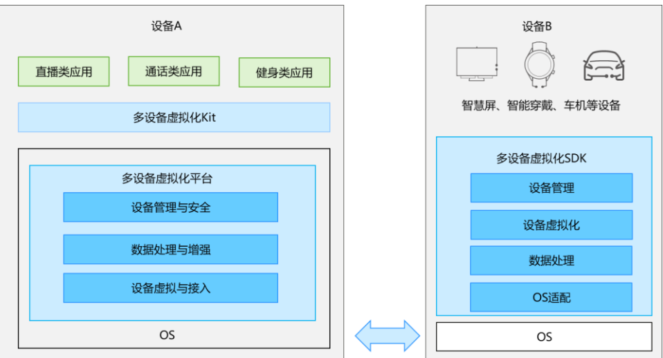
图2-2 分布式设备虚拟化示意图
